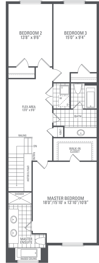
ELEV. 1
