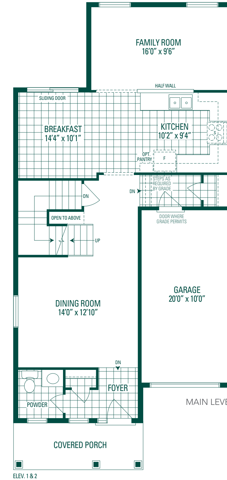
ELEV. 1 & 2
