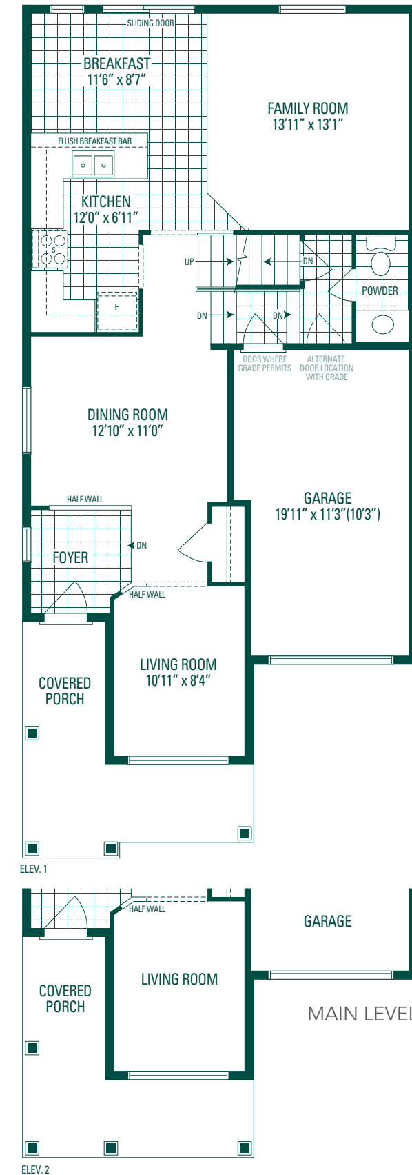
ELEV. 2
